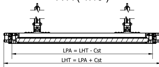
A-A ( 1:10 )
